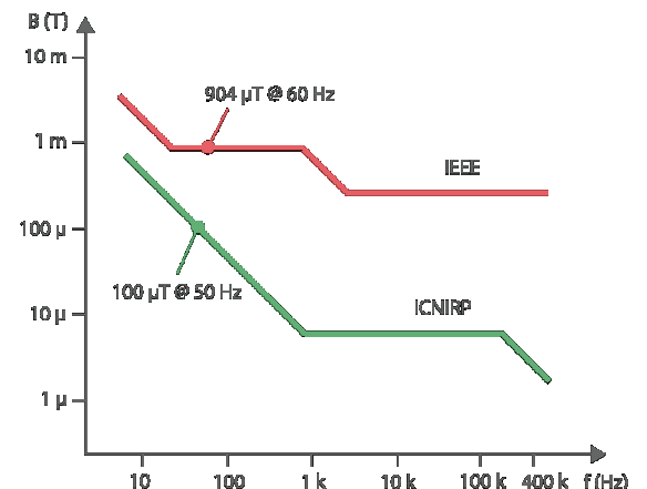
Grenzwertkurven der magnetischen Flussdichte im Frequenzbereich 10 Hz bis 400 kHz nach ICNIRP und IEEE
