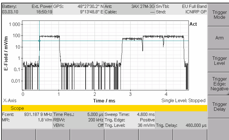
Bild 6: In der Betriebsart Scope zeigt das SRM-3006 die momentane Auslastung der Time Slots innerhalb des TCH.
